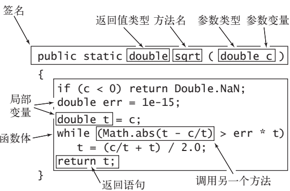
图 1.1.2 静态方法解析
