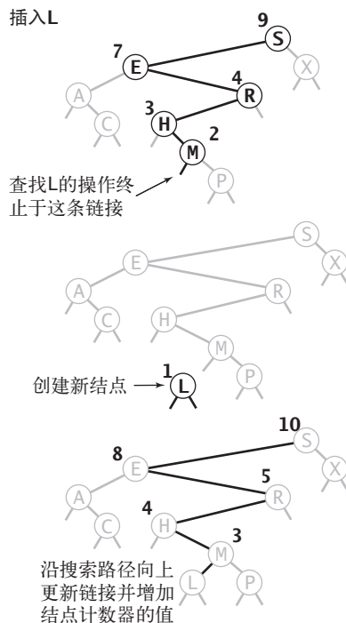
图 3.2.5 二叉查找树的插入操作
