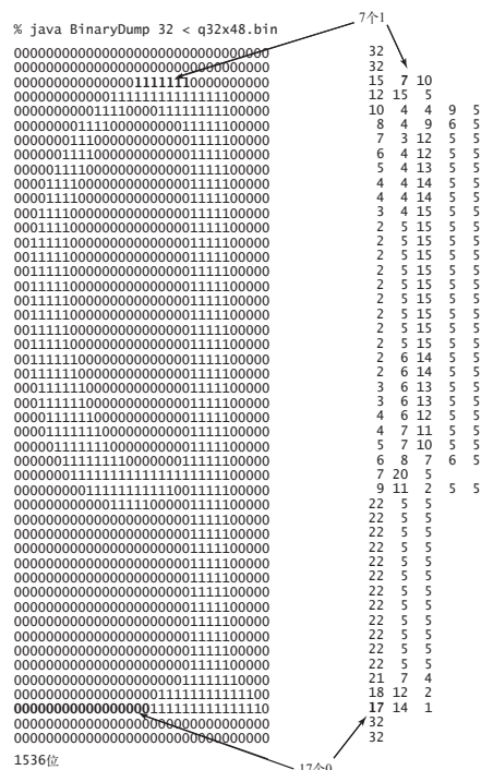
图 5.5.8 一幅典型的位图，每行的游程编码如右所示
