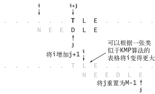
图 5.3.11 Boyer-Moore 算法中的跳跃表的计算
