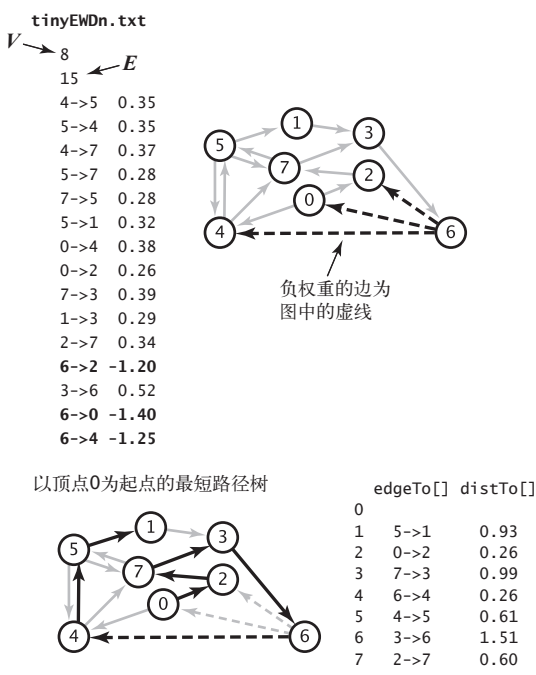
图 4.4.19 含有负权重的边的加权有向图
