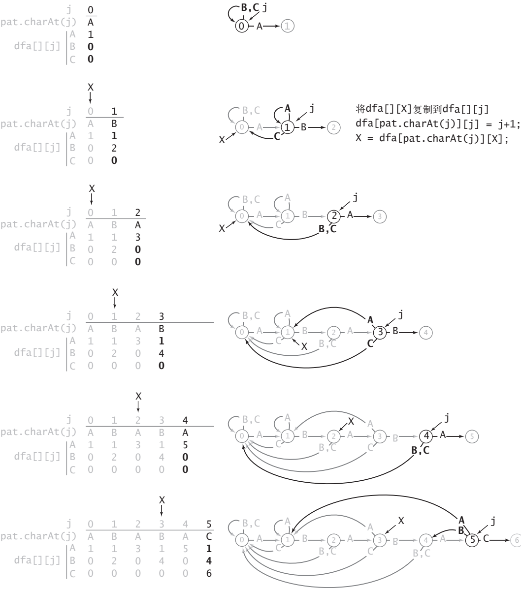
767 图 5.3.9 KMP 子字符串查找算法中模式 A B A B A C 的 DFA 的构造
