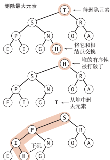
由上至下的堆有序化 (下沉) 的实现
