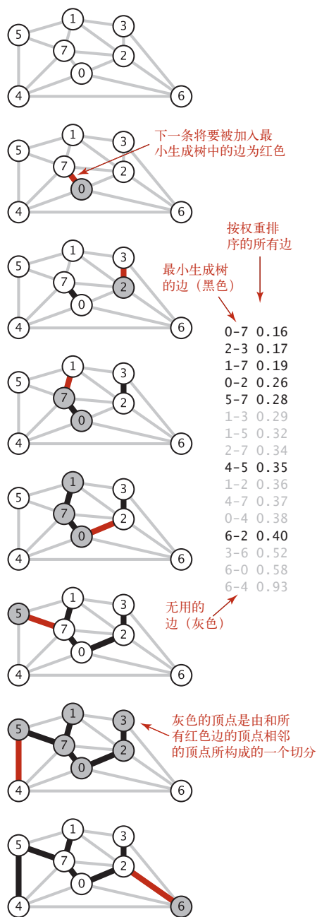
图 4.3.14 Kruskal 算法的轨迹
