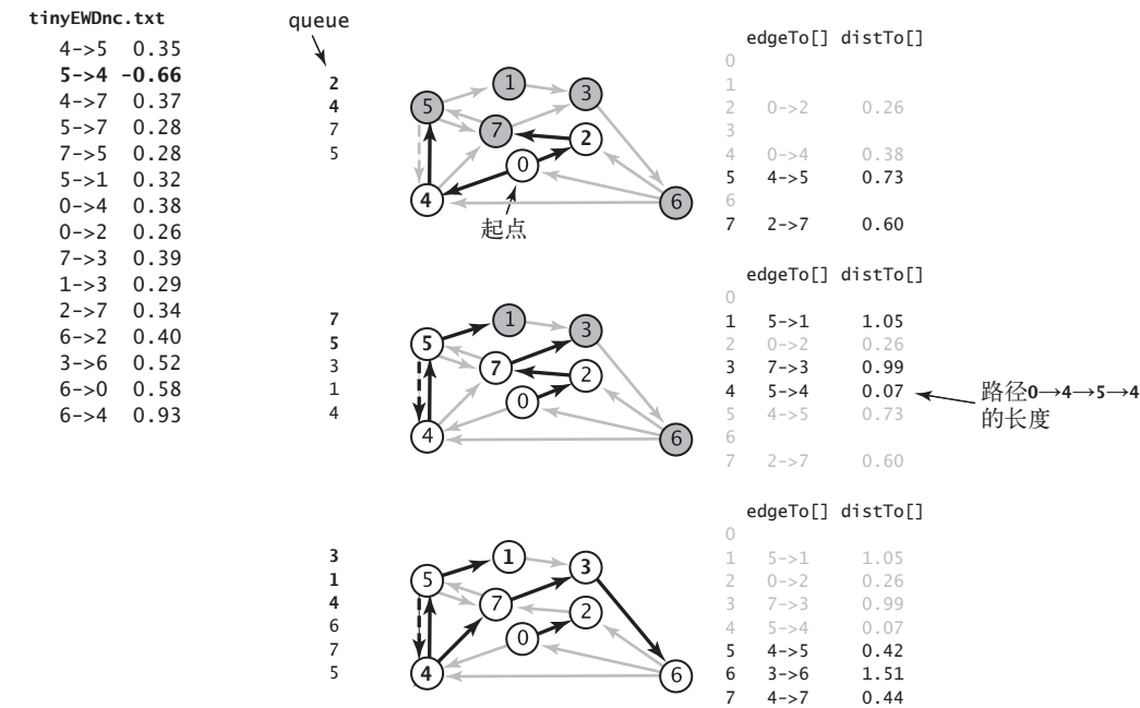
图 4.4.25 Bellman-Ford 算法的轨迹（含有负权重环的图，另见彩插）
