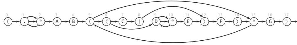
图 5.4.6 模式 (. *AB((C|D*E)F)*G) 所对应的 NFA
