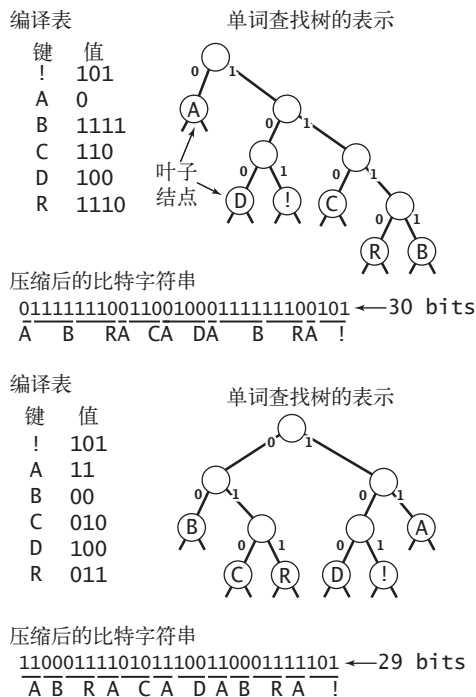
图 5.5.10 两种不同的前缀码
