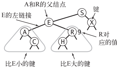
图 3.2.2 详解二叉查找树
